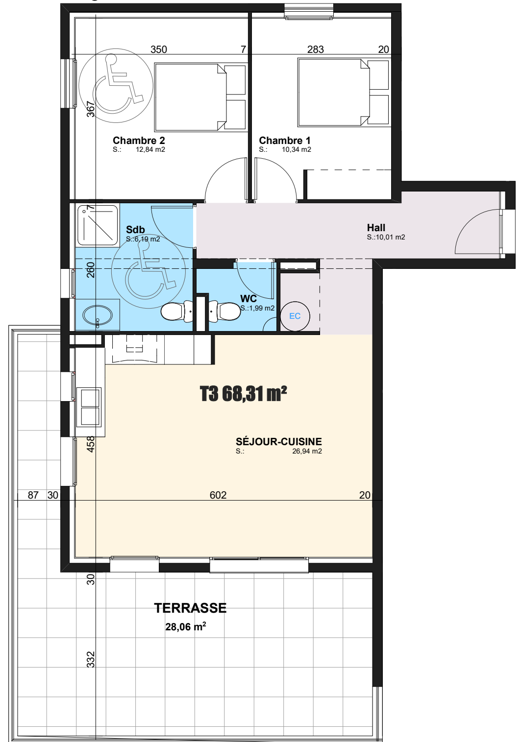
Plan d'étage courant R+2
