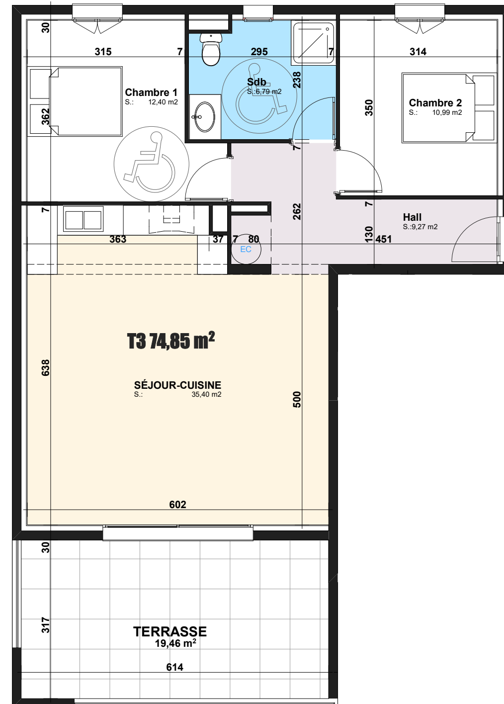
Plan d'étage courant R+1
