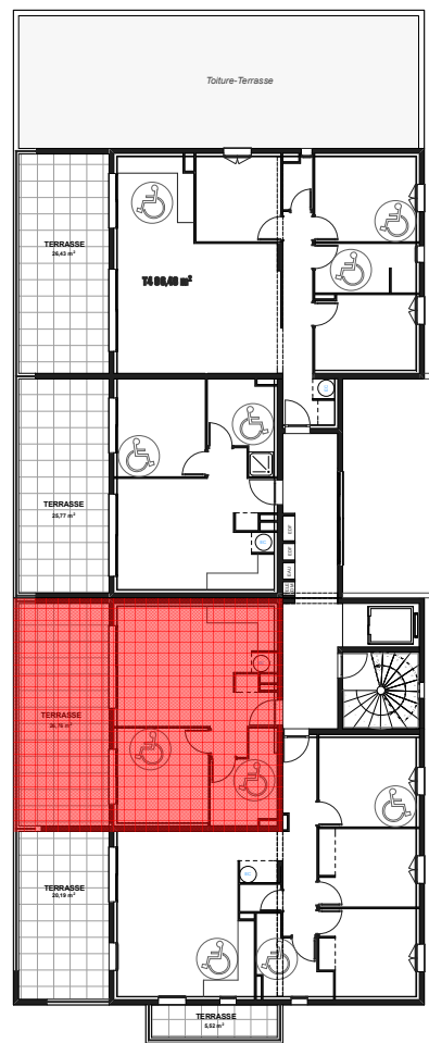
Plan d'étage courant R+1
