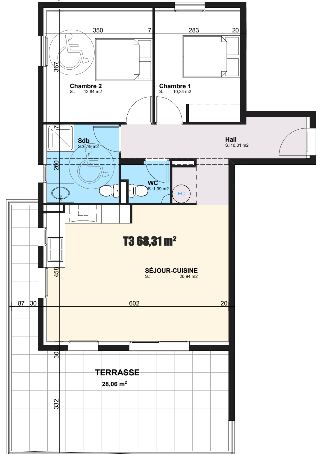
Plan d'étage courant R+3
